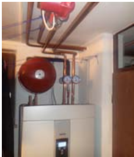
223 litrski hranilnik z avtomatiko za TČ CO 2 ECO.
